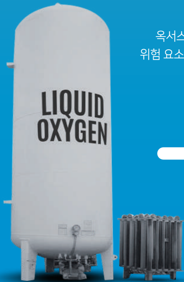
기존 액화 산소가스 매니폴드 시스템
